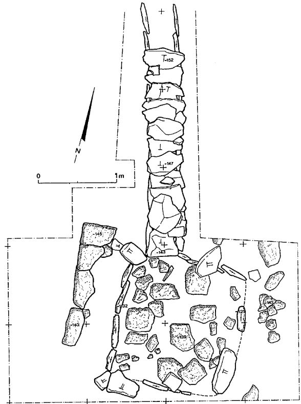
Figura 4 - Plano del temazcal donde se distingue el baño (abajo) y el drenaje de laja (arriba).
